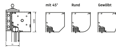
RS Smart 100 Eckig
