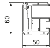
Führungsschienen
