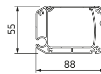
Ausfallprofil
